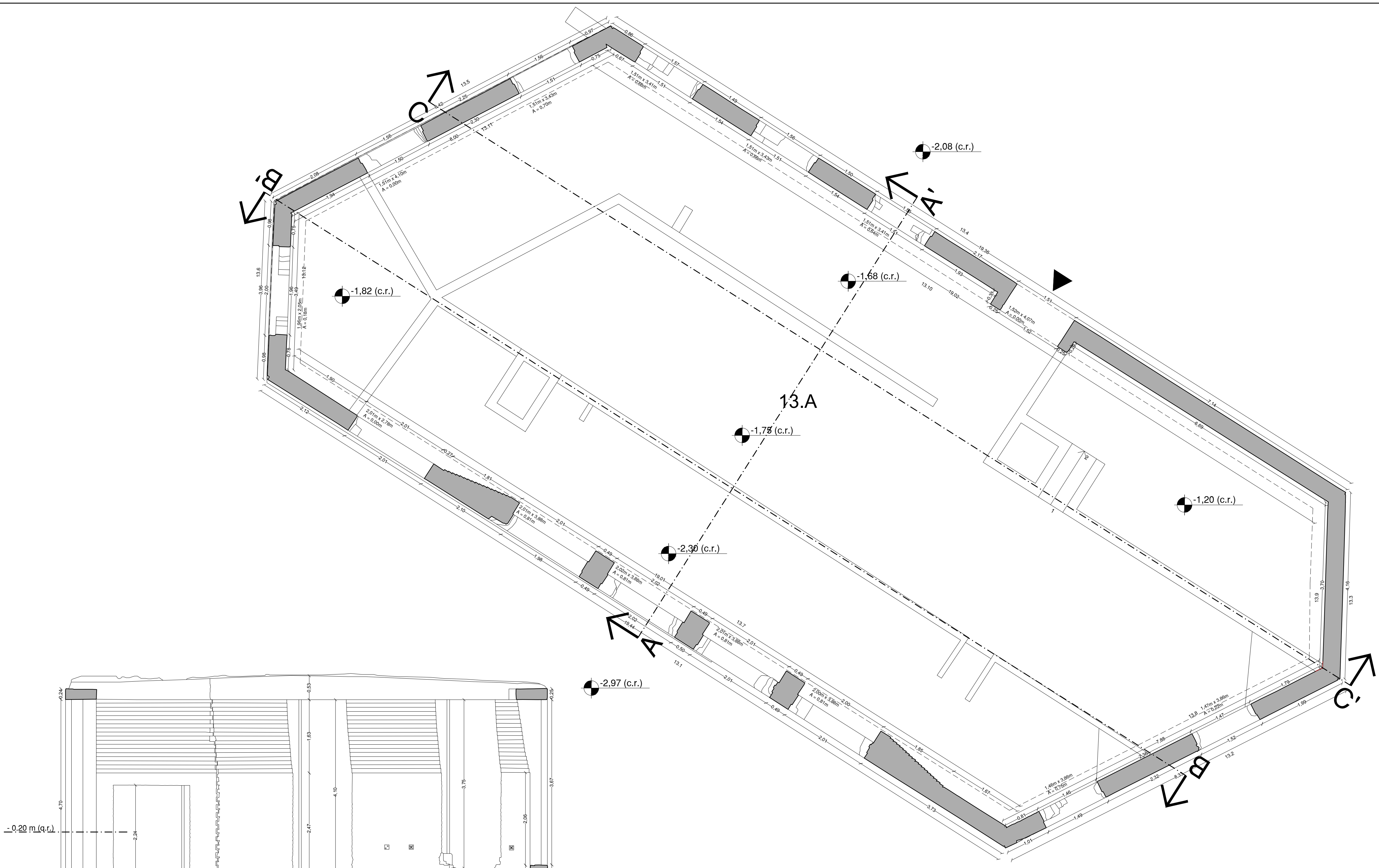
Planta a cota -0,02 (c.r.)
