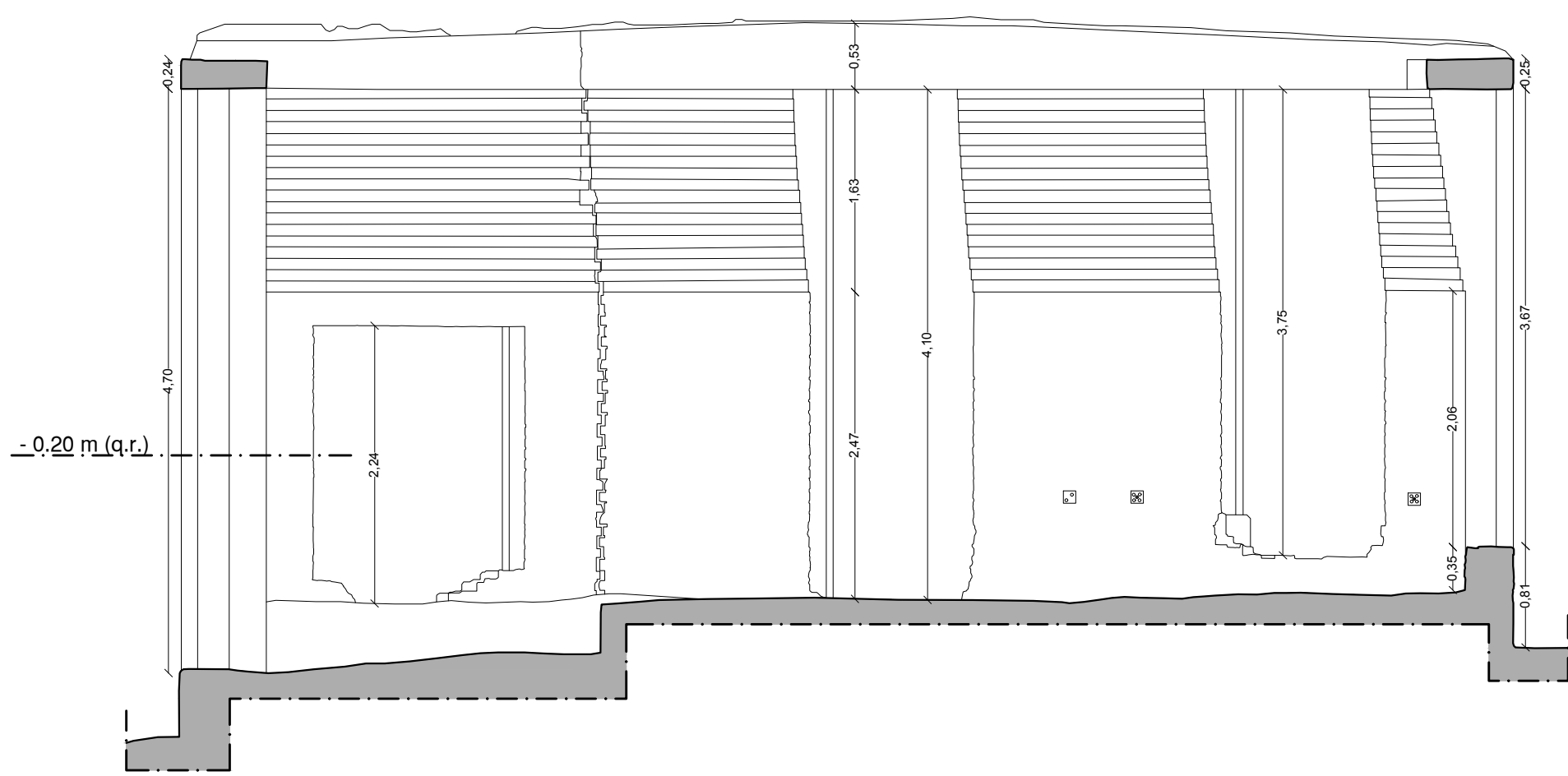
Sección A-A'
