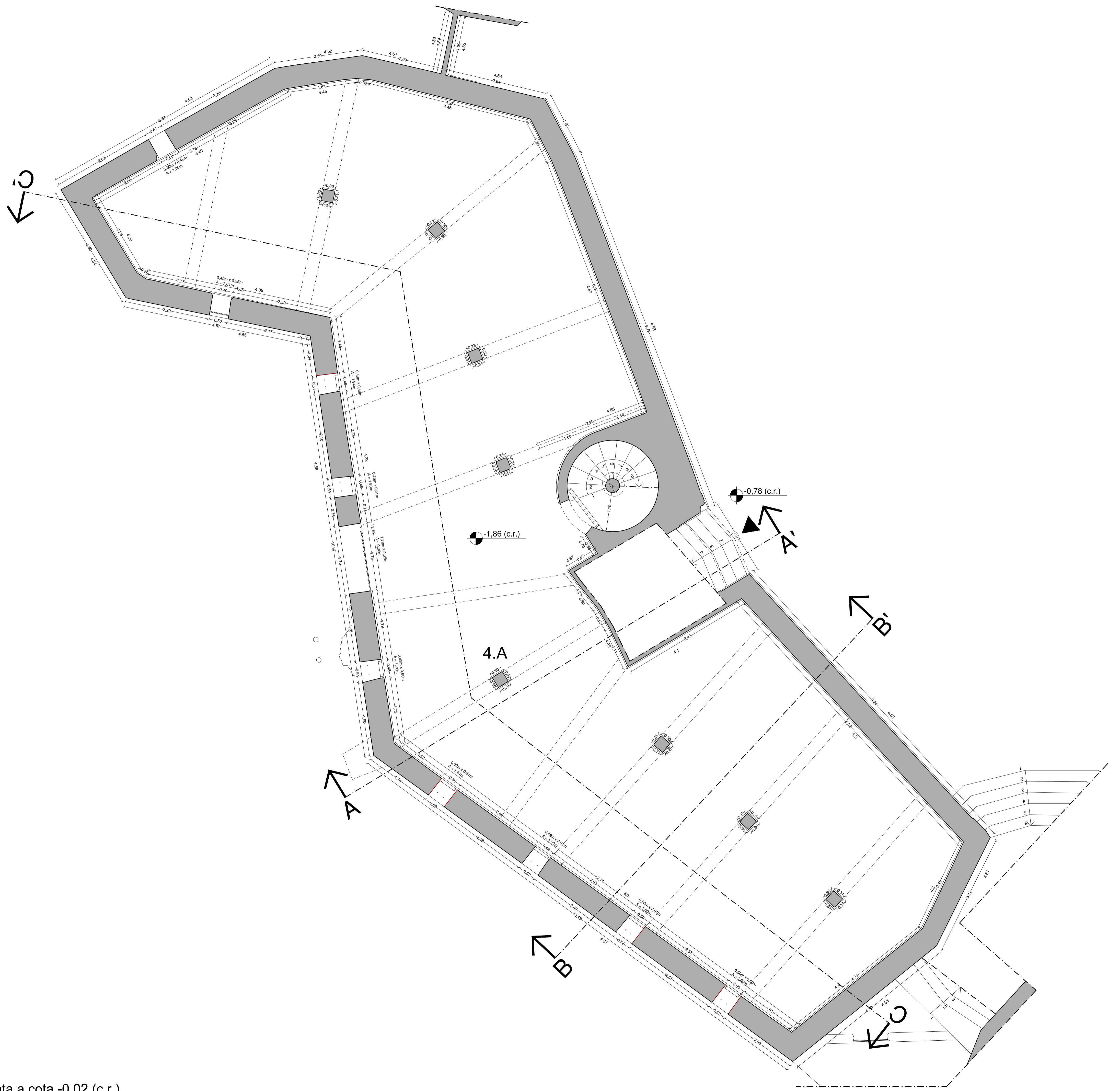
Planta a cota -0,02 (c.r.)
